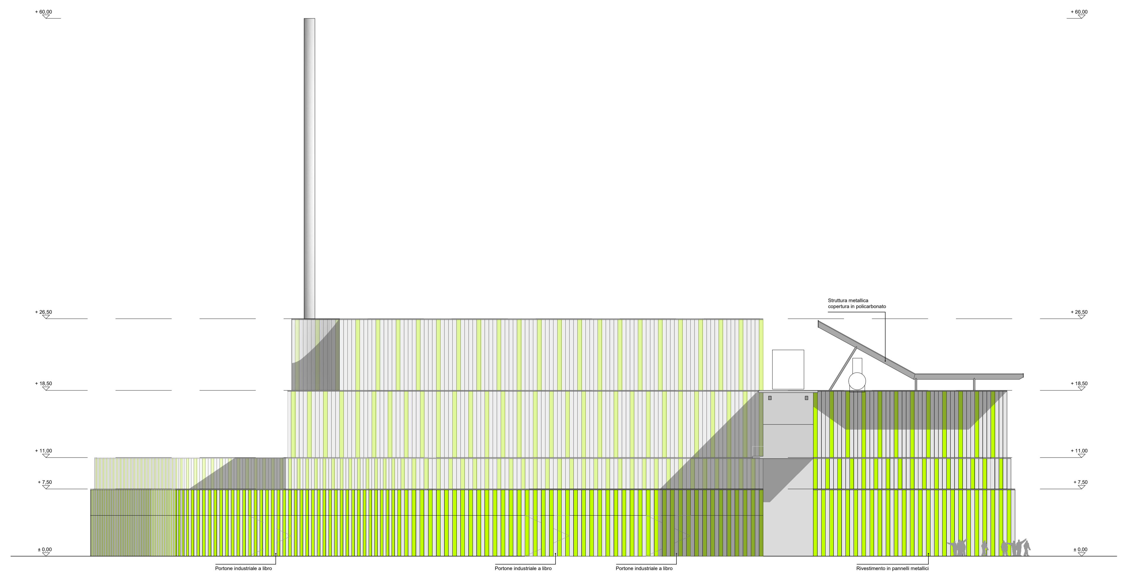
PROSPETTO EST
